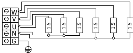
DRFT6-90NS-CNR 9,0 kW
