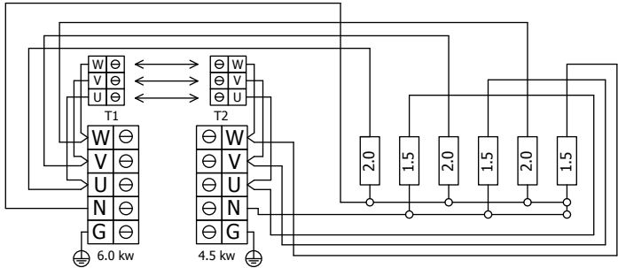
DRFT6-105NS-CNR 10,5 kW
