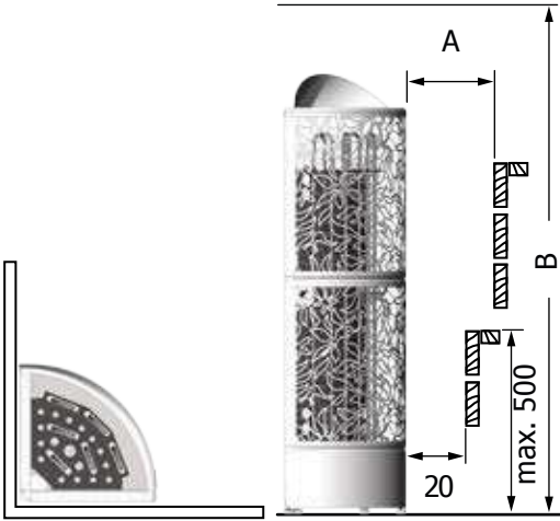
Kuva 2 Fig. 2 Vähimmäisetäisyydet (mm) Minimum safety distances (mm)
