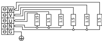
DRFT6-80NS-CNR 8,0 kW
